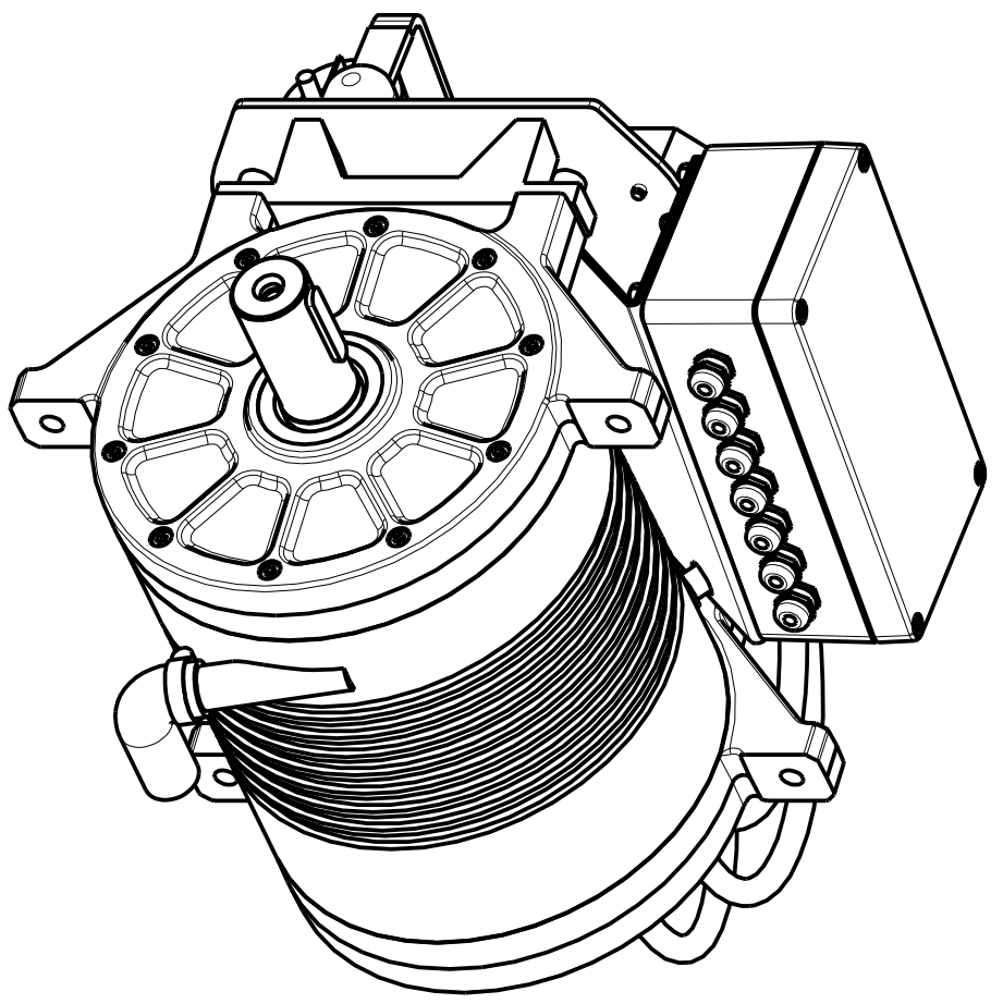
Körvonalrajz 15kW-os 1450 1/min névleges fordulatszámú permanens mágneses motorhoz
