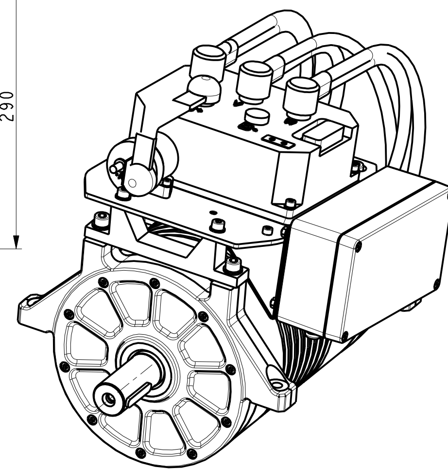
Körvonalrajz 15kW-os 1450 1/min névleges fordulatszámú permanens mágneses motorhoz
