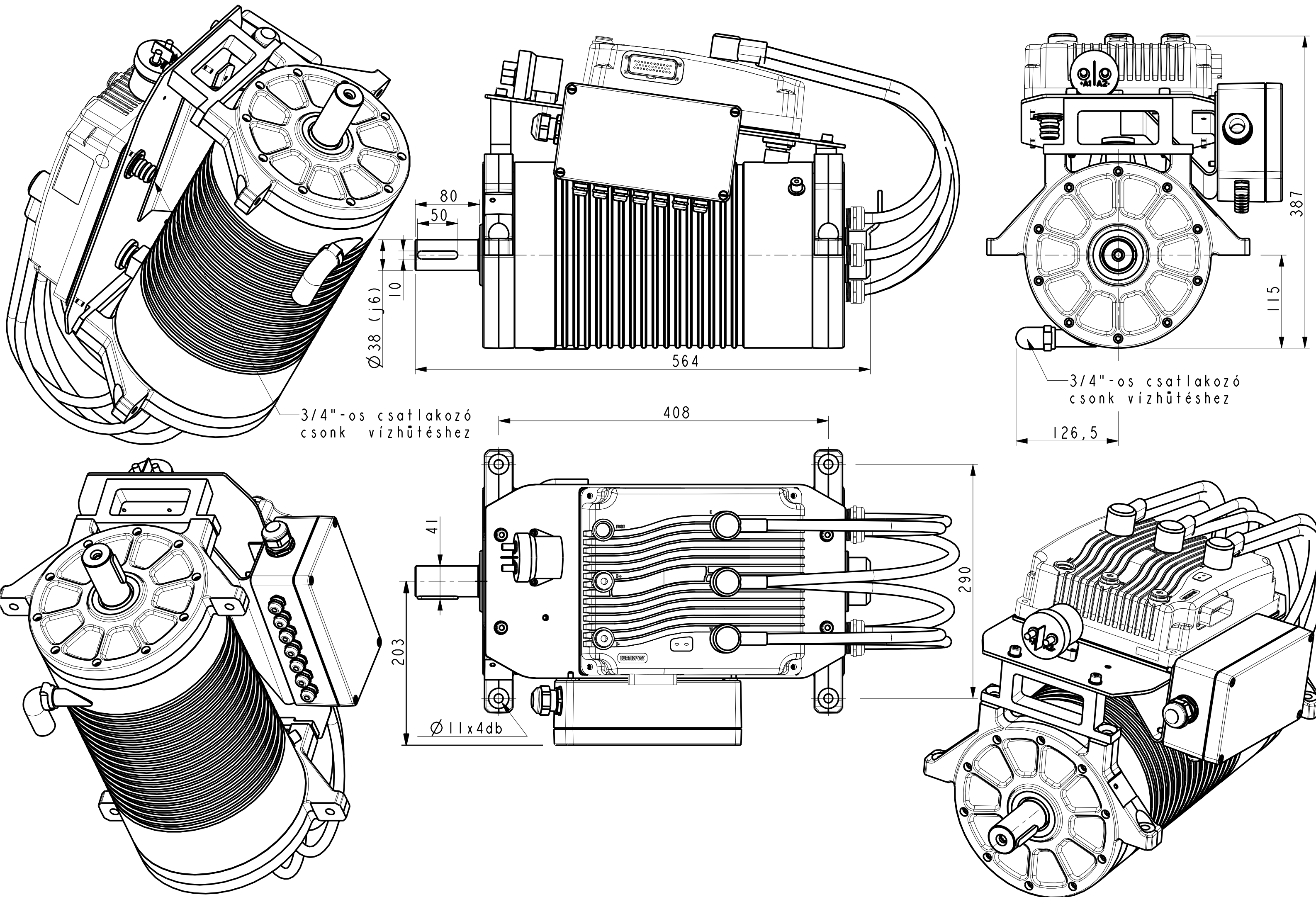
Körvonalrajz 40kW-os 2000 l/min névleges fordulatszámú permanens mágneses motorhoz RevB
